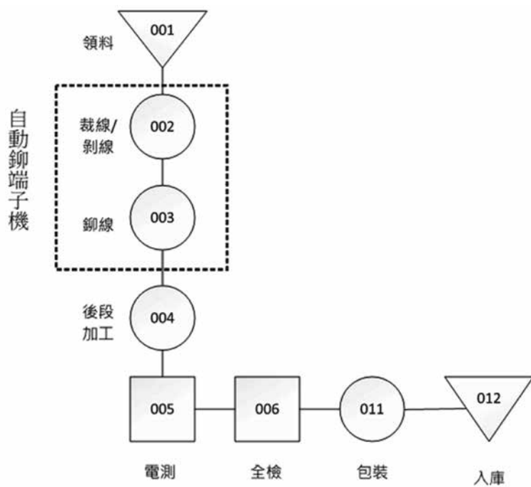
產製流程圖
