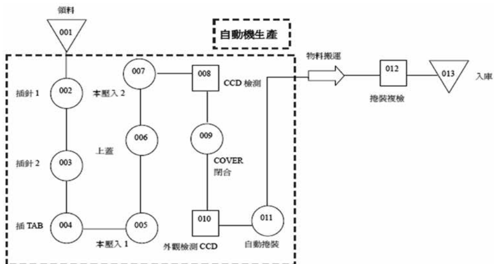
產製流程圖
